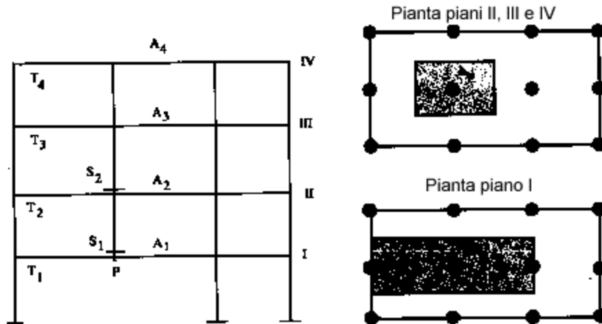
Esempi schematici di individuazione dell'area di spettanza per la determinazione del coefficiente di riduzione dei carichi.
