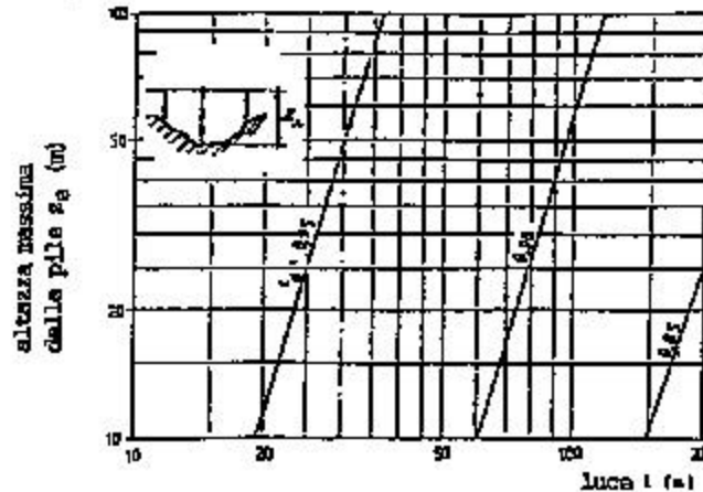
Fig. C.7.12. - Ponti stradali, ferroviari e pedonali
