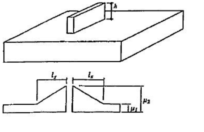
Coefficienti di forma in corrispondenza di parapetti e pareti verticali.
