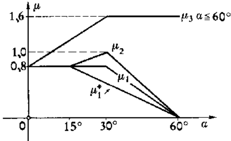
Coefficienti di forma per coperture a falde
