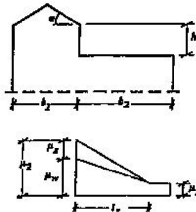
Coefficienti di forma per bruschi cambiamenti di quota
