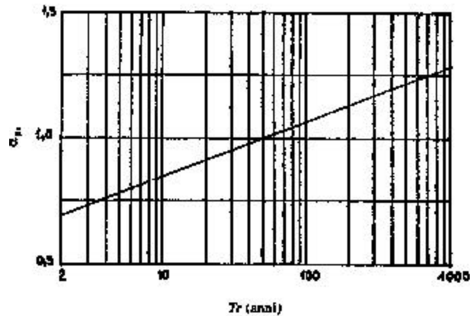
Valori dell'azione del vento in funzione dell'intervallo di ritorno
