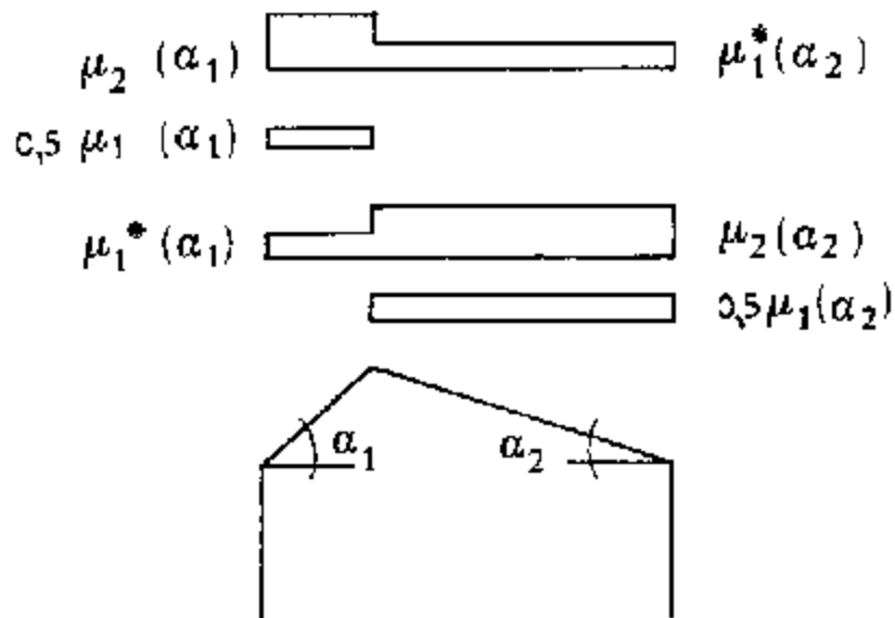
Condizioni di carico per coperture a due falde
