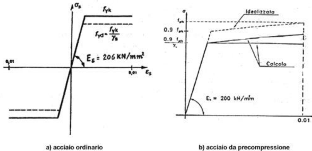
Diagramma di calcolo \sigma-\epsilon
