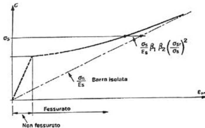
Diagramma \varepsilon_{sm} - \sigma_s
