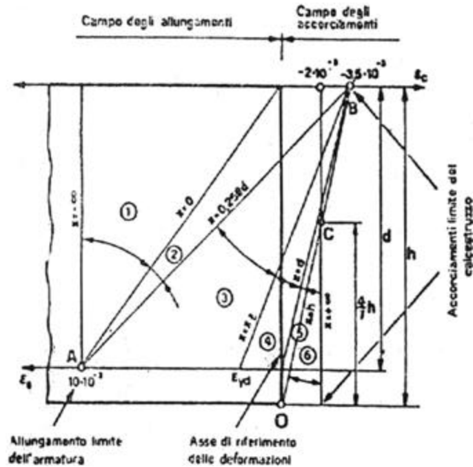
Diagramma di deformazione allo stato limite ultimo
