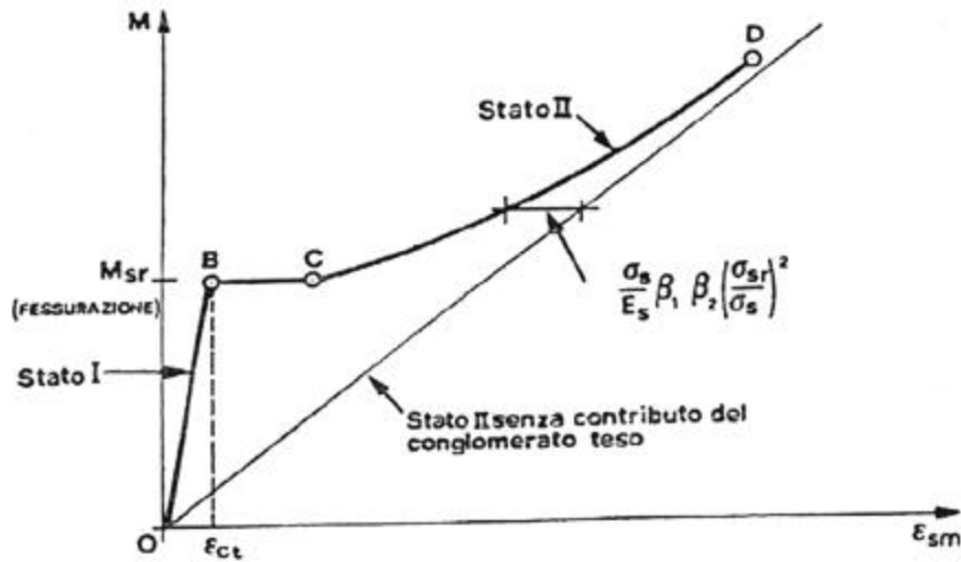
Diagramma M - \epsilon_{sm}
