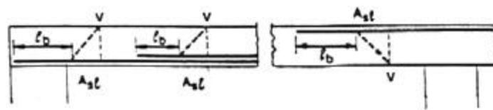
Fig. 3-1 per l_b , lunghezza di ancoraggio, vedasi punto 5.3.3.
